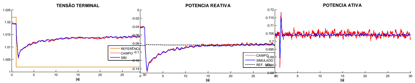
Figura 1 - Exemplo de Validação de um Modelo - Resposta do UEL
