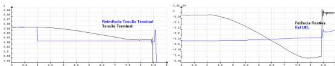
Figura 7 – Ensaio Real de Campo – Atuação do Bloqueio do Relé 40 no Ensaio do UEL Somador
