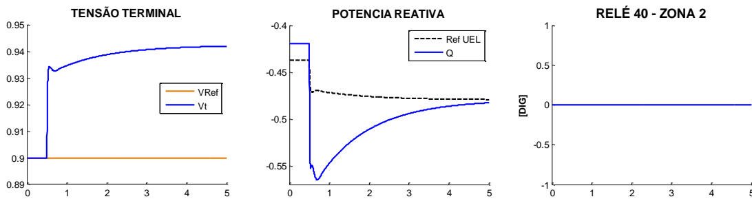
Figura 12 – Simulação Aumentando a Folga da Coordenação Estática
